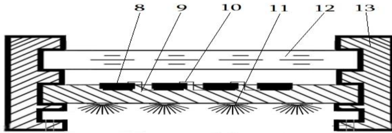
Նկ.3. Արևային էներգիայի կերպափոխման ֆոտովոլտային մոդուլի կառուցվածքի ու շրջանակի ակոսների հատույթները և կապակցող շերտին կապված այլումինե թաղանթների փնջերը
