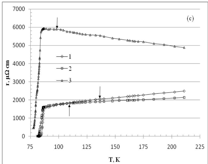
Նկ. 1. Տեսակարար դիմադրության ( r ) ջերմաստիճանային կախվածությունը 1, 2 և 3 նմուշների համար ջերմաստիճանային տարբեր տիրույթներում (a, b, c): Ուղղահայաց սլաքները մատնանշում են համապատասխան նմուշներում փսնդոգոտիական ռեժիմի առաջացման ջերմաստիճանները ( T^p ):
